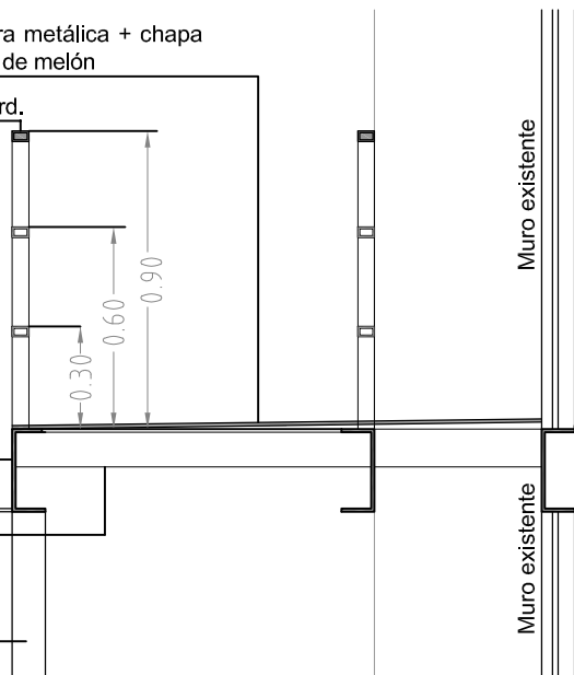
Corte de baranda
